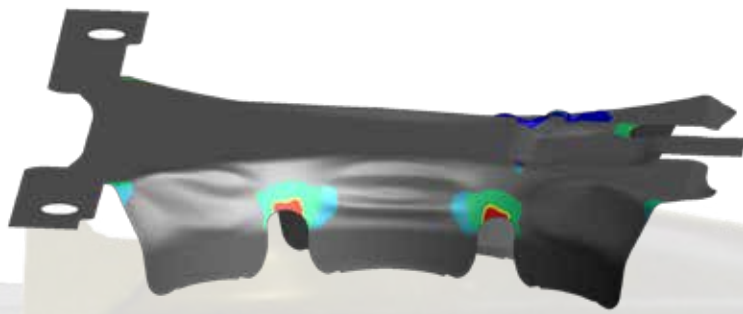
Vorhersage der Risse und Falten mit Stampack
