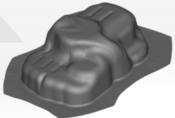
Vorhersage der Faltenbildung durch eine Simulation mit Stampack
