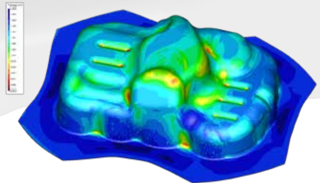
Vorhersage der Ausdünnung durch eine Simulation mit Stampack
