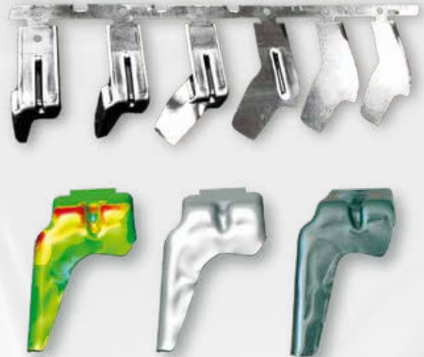
3D Volumensimulation ermöglicht die genaue Simulation des Umformprozesses: Realität (rechts) und Simulation (Mitte) sind praktisch nicht zu unterscheiden.
