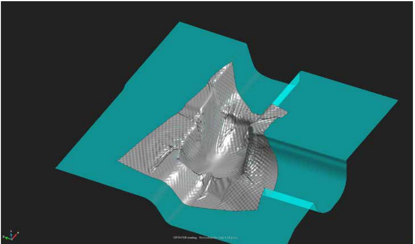
Mit Stampack Xpress simuliertes Prägeteil.
