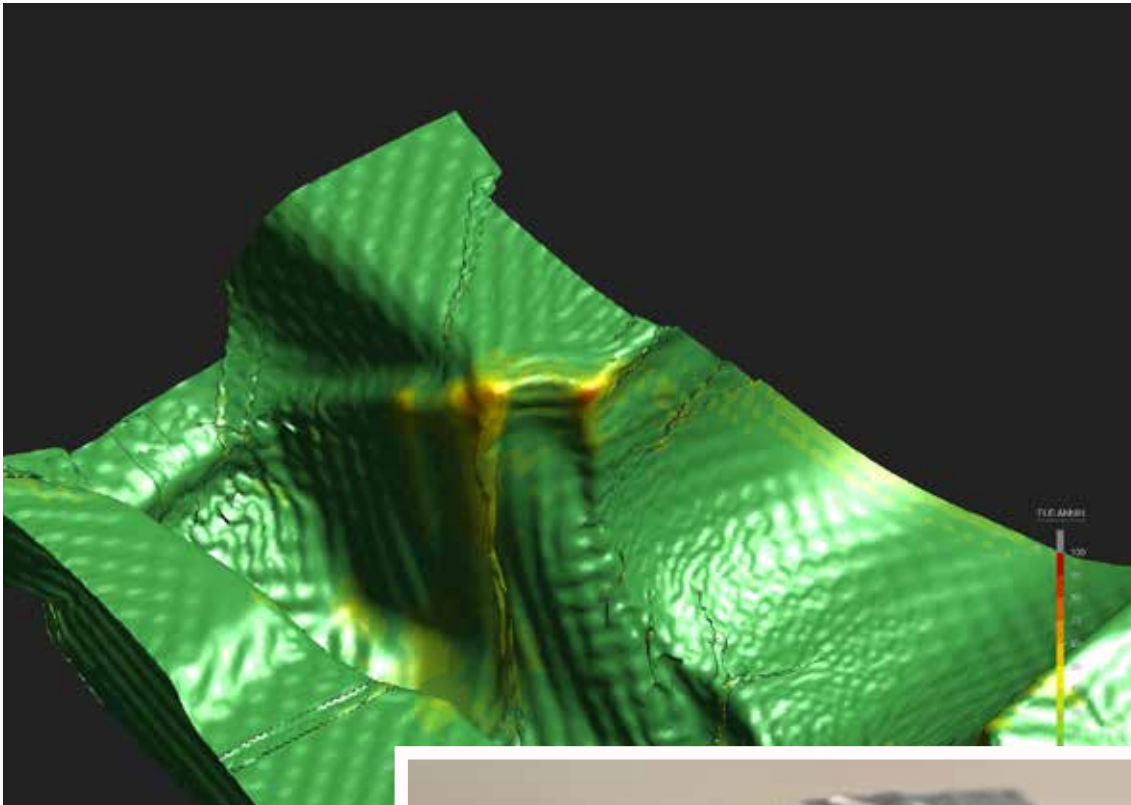
Faltenverlauf und Materialbeanspruchung einer geprägten Schale aus 1.4541 mit einer Blechdicke von t = 0,15 mm.
